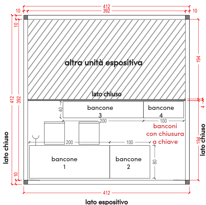
PIANTA
