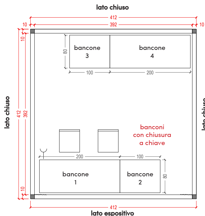
PIANTA
