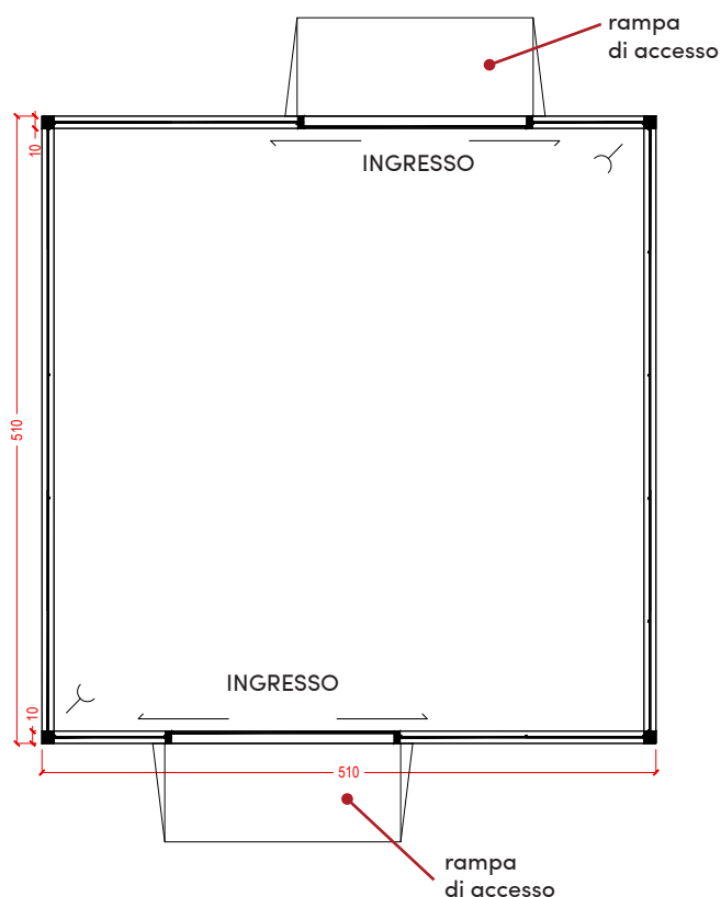
PIANTA
